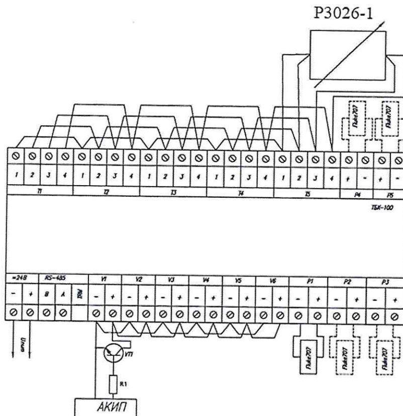
Рисунок 1 – Схема подключения средств поверки к ИК температуры, давления, расхода VT1 – транзистор КТ3102 или аналогичный, R1 – резистор, номинальное сопротивление 10 кОм, номинальная мощность не менее 0,125 Вт
