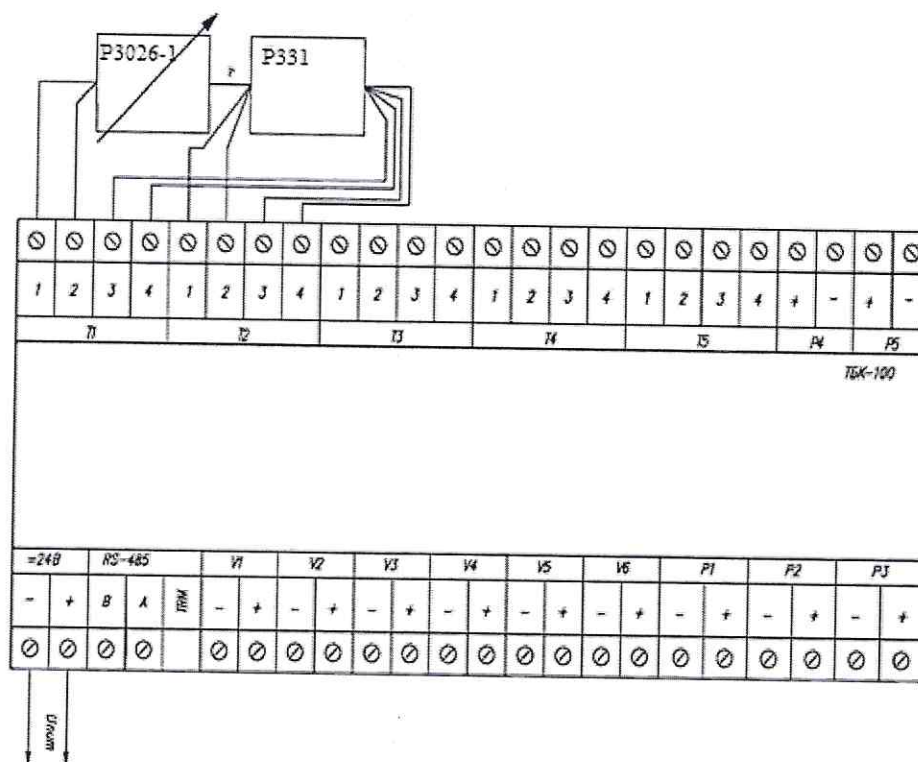
Рисунок 2 – Схема подключения средств поверки к ИК разности температуры Р – перемычка, выполненная многожильным медным проводом сечением не менее 2,5 \text{ мм}^2 и длиной не более 300 мм
